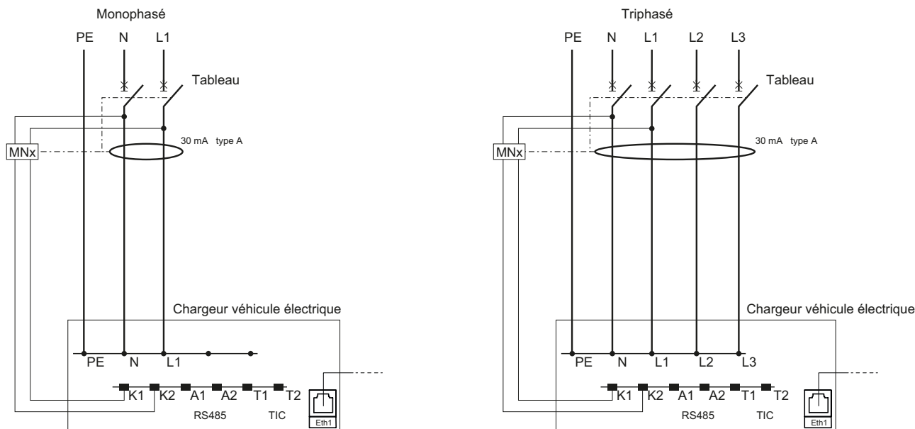
Déclencheur à minimum de tension (MNx)
