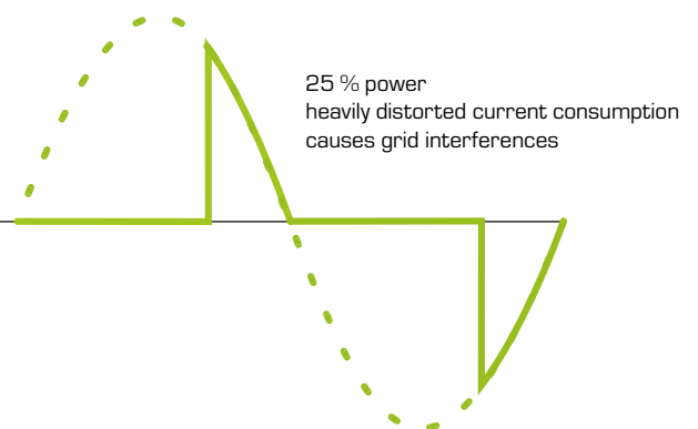
Thyrisor
