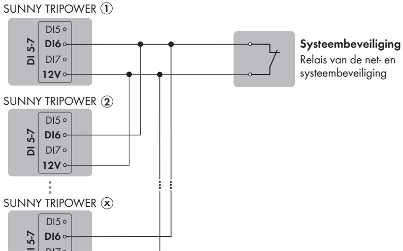
Afbeelding 13: Aansluiting van een relais voor de externe net- en systeembeveiliging aan de digitale ingang DI 6
