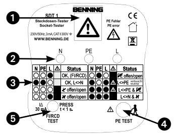
Obr. 1.: Čelní strana přístroje
