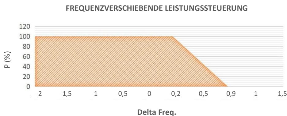
Beispiel einer PV-Wechselrichterfunktion, die Leistung und Deltafrequenz zeigt
